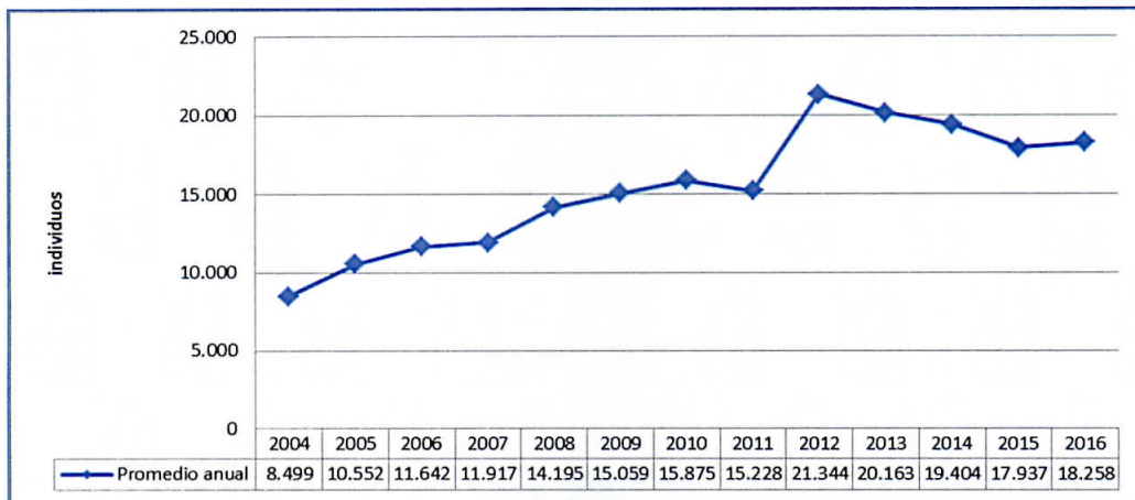
Gráfico N° 1: Promedio Anual abundancia de las tres especies de Flamencos en el Salar de Surire Período 2004 - 2016
