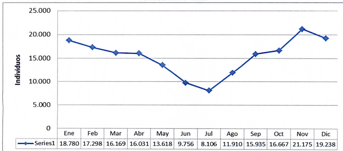
Gráfico N° 2: Promedio anual mensual abundancia de las tres especies de flamencos en el Salar de Surire Período 2004 - 2016
